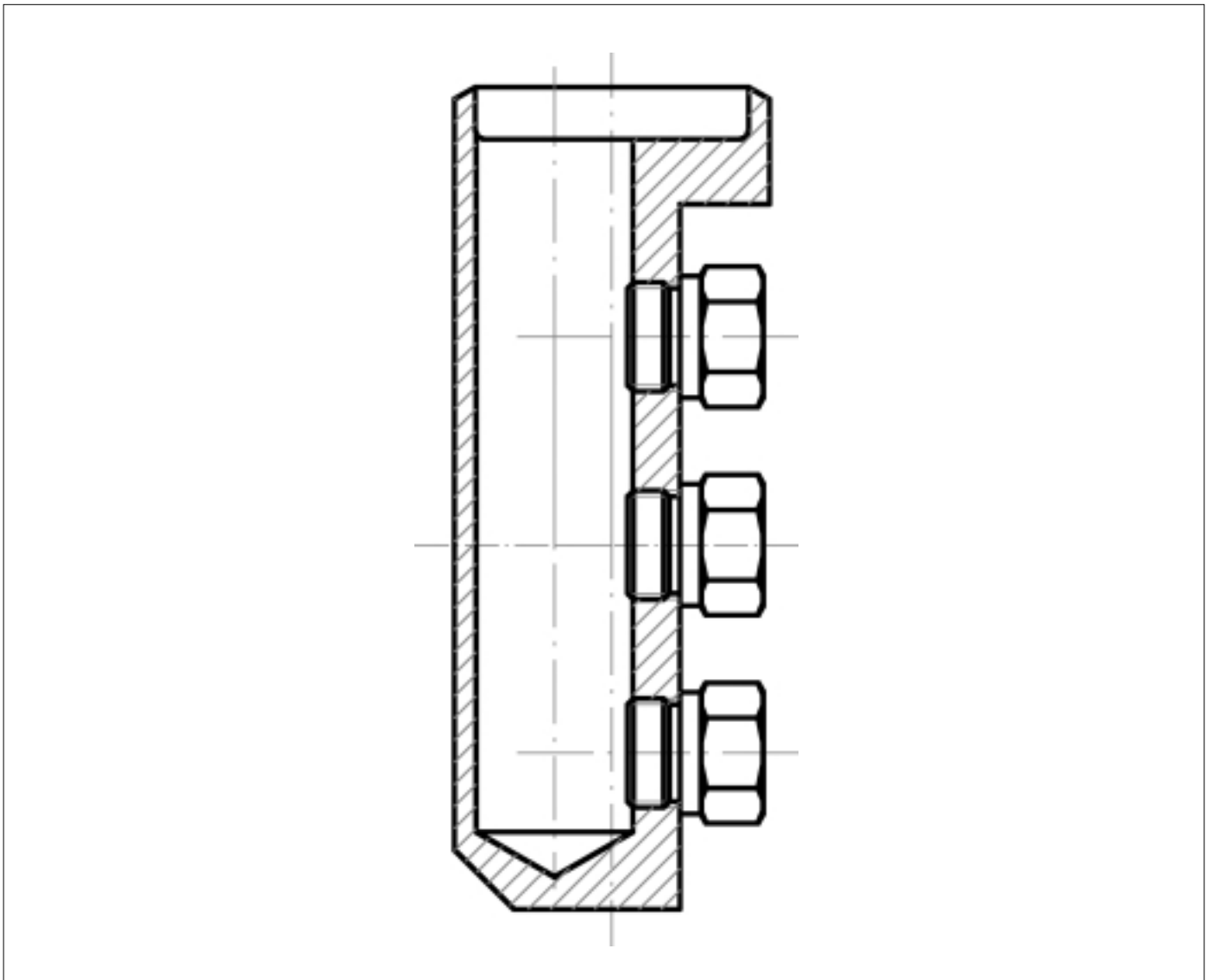
Düsen durch Heftnaht gesichert
